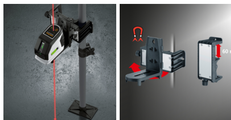
Optional: CombiRangeXtender 40 Artikel-Nr. 033.35A
